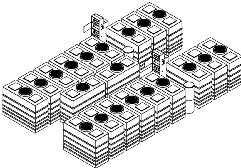
Abbildung 1: Grauwasser-Recycling-Anlage GWI 55.2 – 55.000
