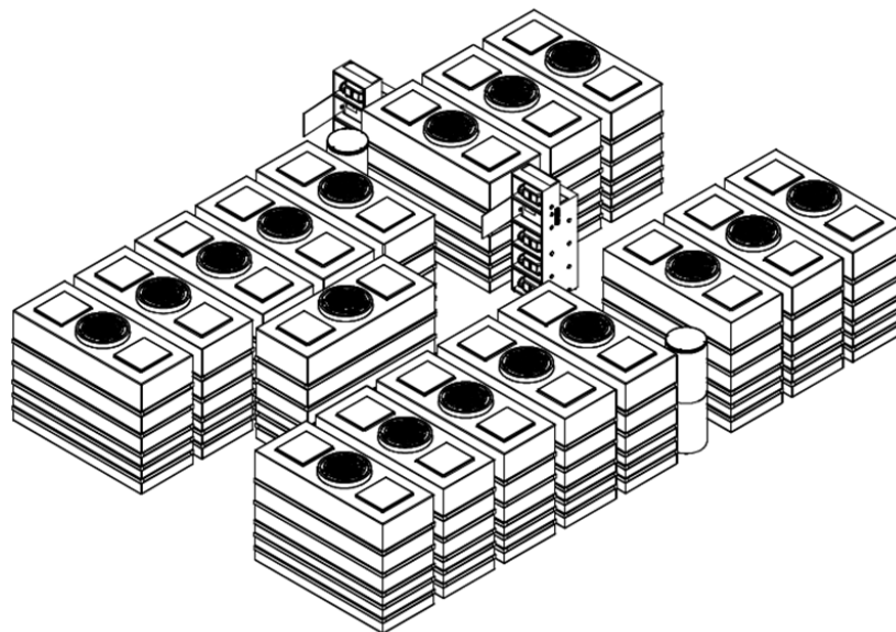
Abbildung 1: Grauwasser-Recycling-Anlage GWI 45.2 – 45.000
