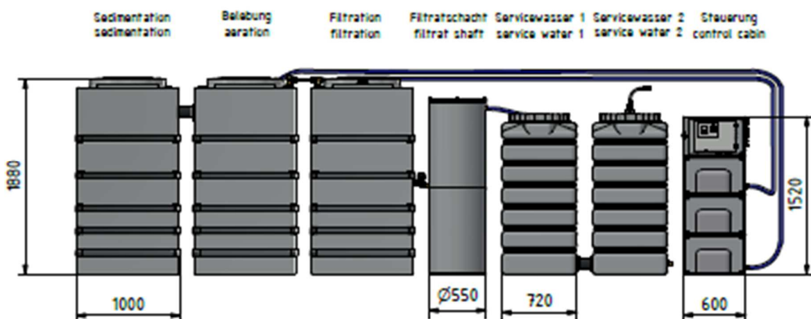
Abbildung 1: Grauwasser-Recycling-Anlage GWI 6.2 – 6.000
