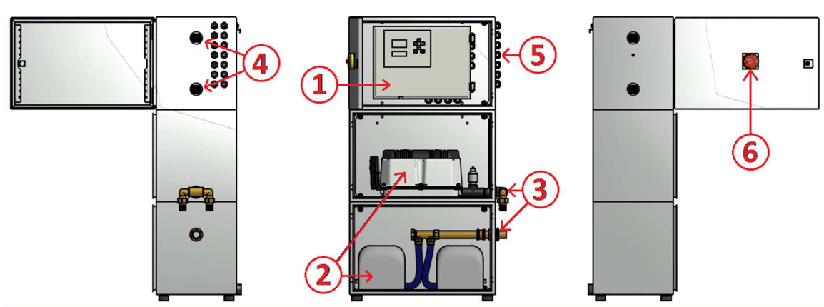
Abbildung 2: Steuerschrank (variable)
