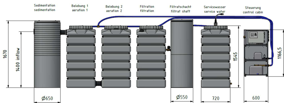
Abbildung 1: Grauwasser-Recycling-Anlage GWI 2.3 – 2.000
