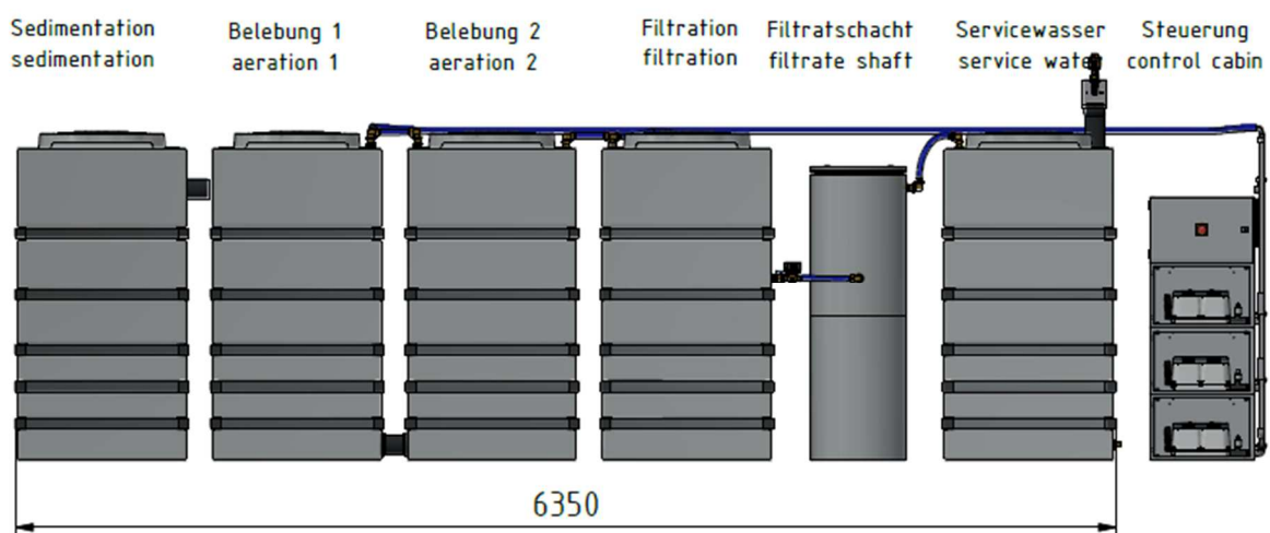
Abbildung 1: Grauwasser-Recycling-Anlage GWI 10.2 – 10.000
