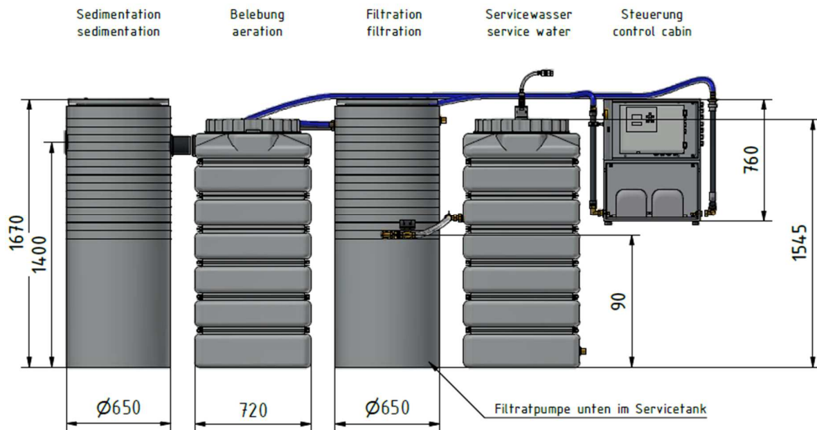
Abbildung 1: Grauwasser-Recycling-Anlage GWI 1.3 – 1.000
